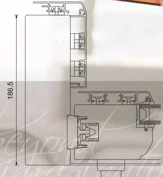
Horizontalni presek
