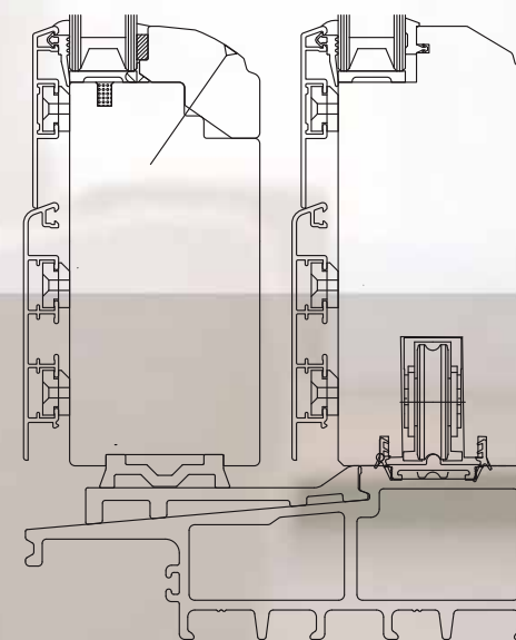
Vertikalni donji presek
