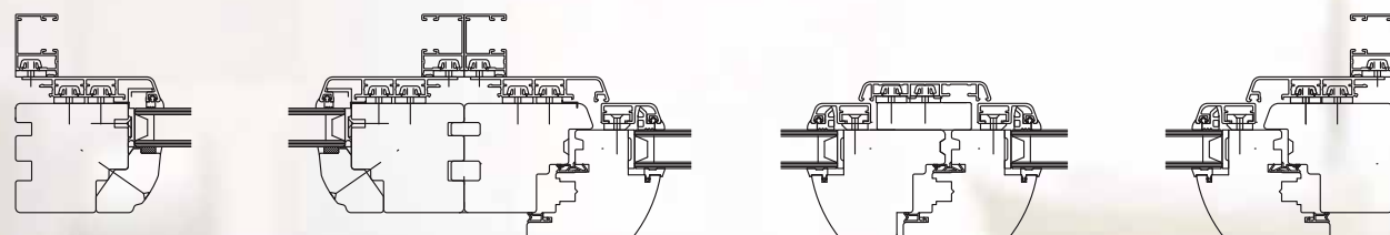
Horizontalni presek drvo - aluminijum (dvokrilni prozor sa fiksom)
